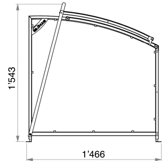
Seitenansicht offen
